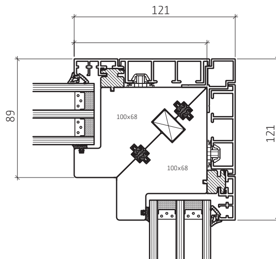
Schmale Ecke
