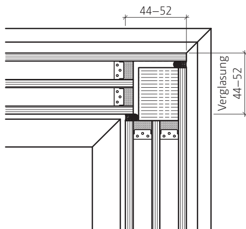
Ganzglasecke
