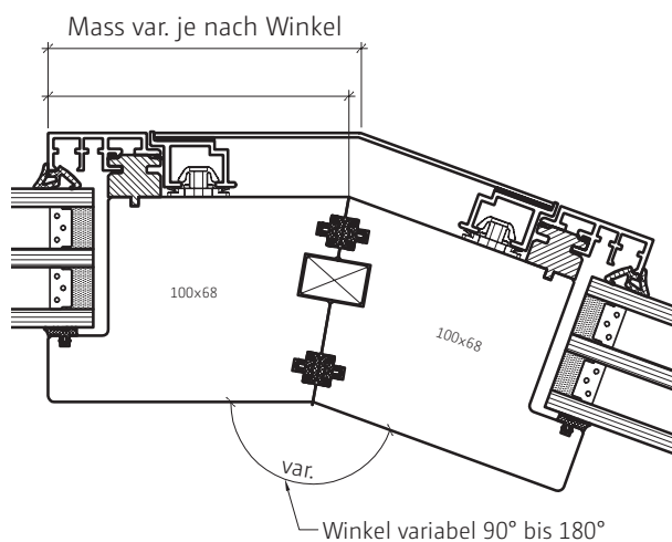
Variable Ecke
